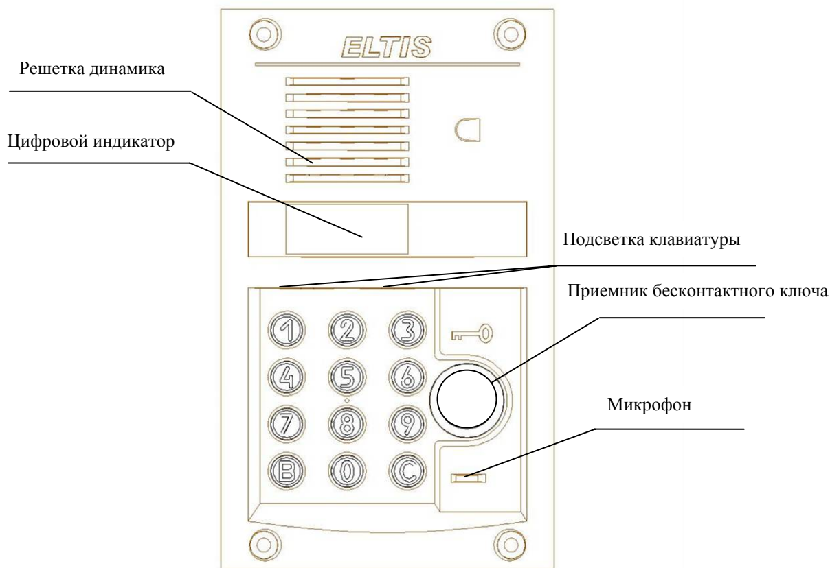
Рис.1 Внешний вид со стороны лицевой панели блока вызова DP300-RD24.
